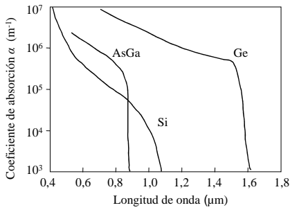
Fig. 2.5. Coeficiente de absorción óptica de diferentes semiconductores.
